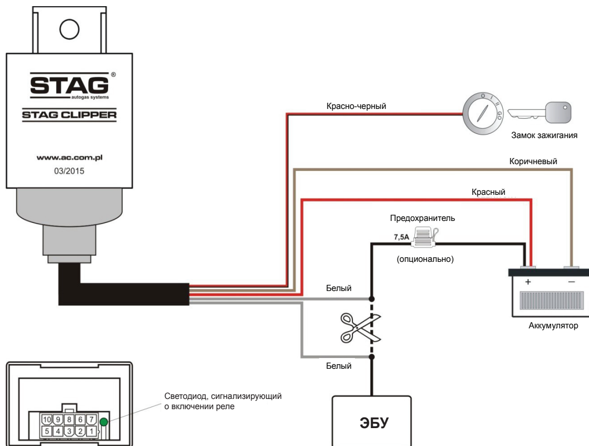
Сх. 1. Схема подключения эмулятора STAG Clipper к проводке автомобиля.
