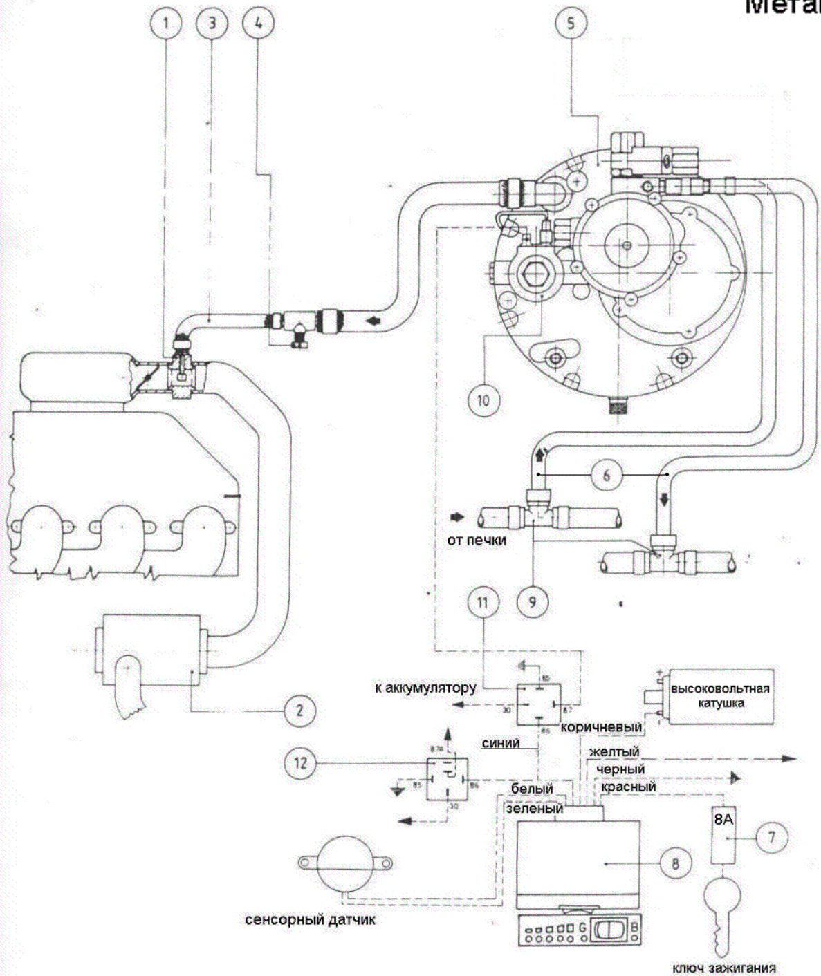
Схема подключения электронного редуктора М91 на автомобиль с инжектором
