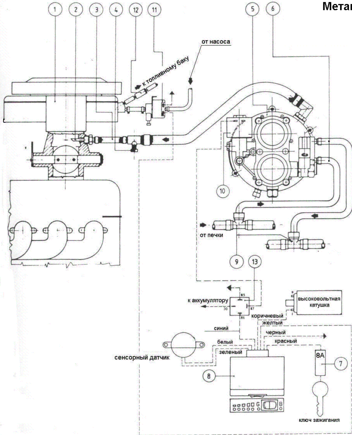
Схема подключения электронного редуктора M96/97 на автомобиль с карбюратором
