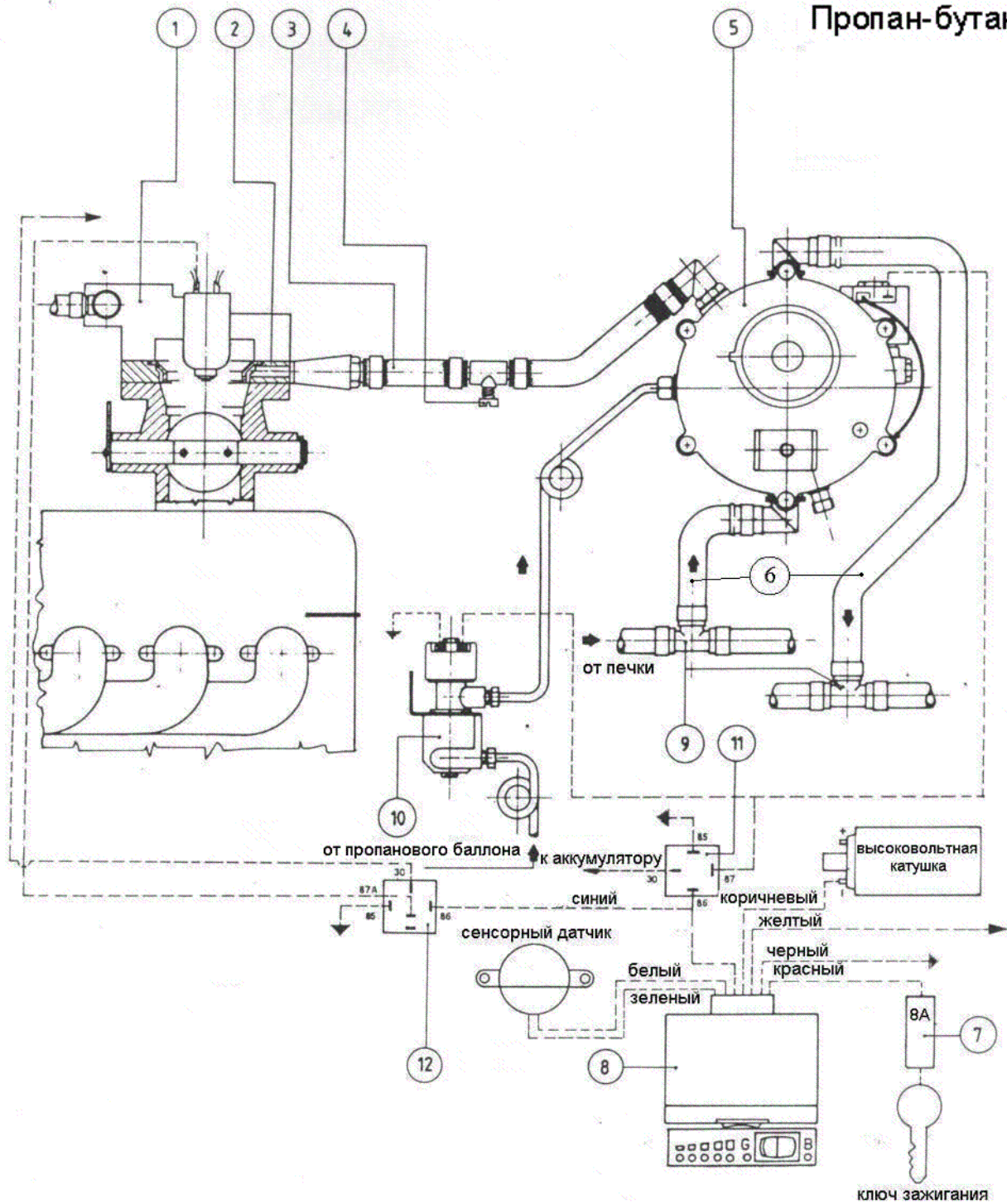
Схема подключения электронного редуктора М84 на автомобиль с моноинжектором
