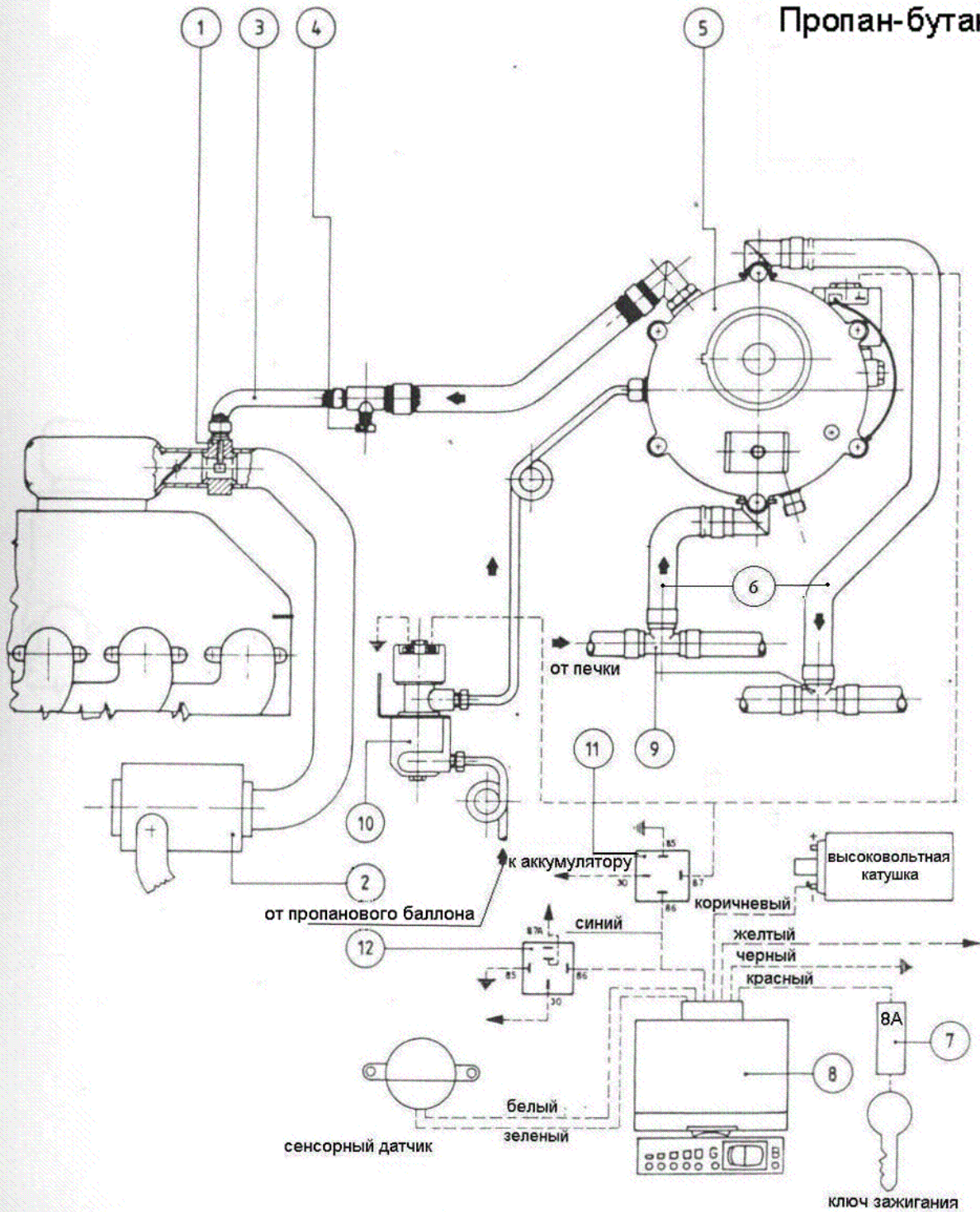
Схема подключения электронного редуктора M84 на автомобиль с инжектором
