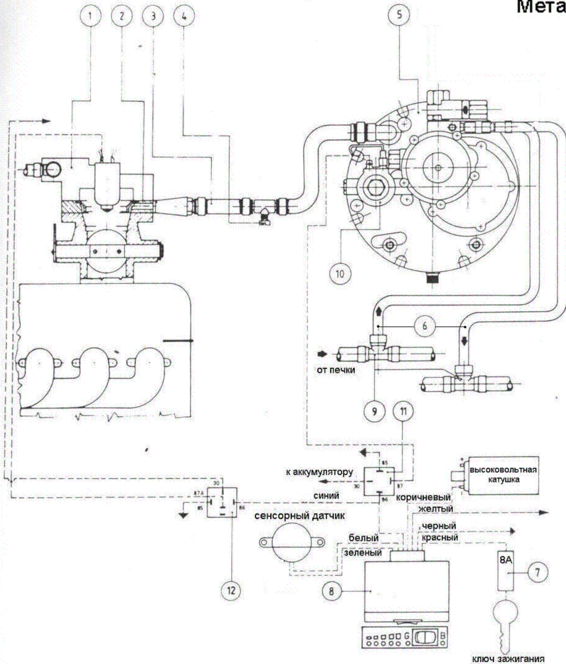
Схема подключения электронного редуктора М91 на автомобиль с моноинжектором
