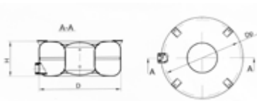
Zbiorniki toroidalne zewnętrzne pełne
