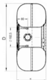
Zbiorniki toroidalne pionowe
