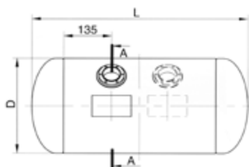
Zbiorniki walcowe
