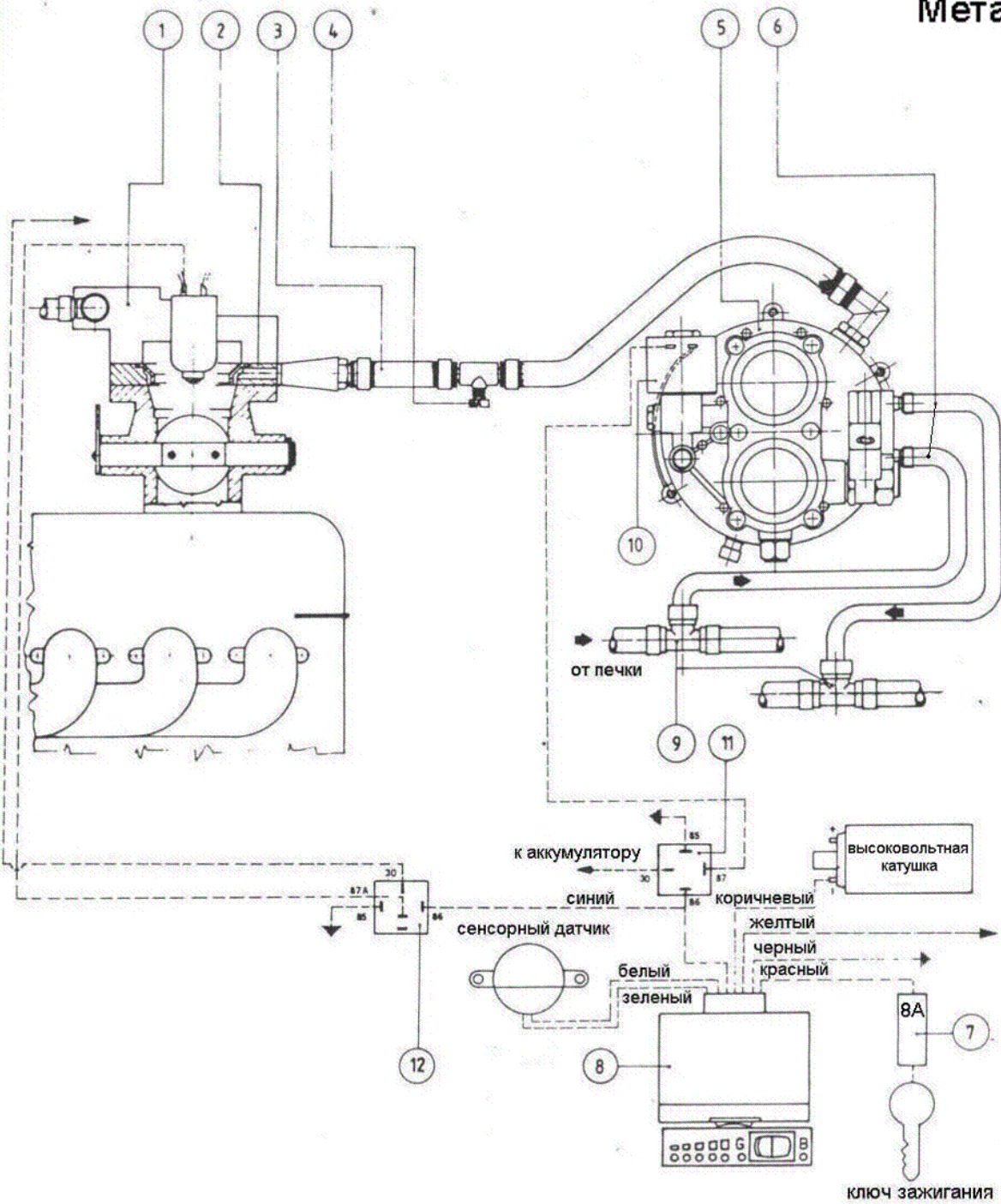
Схема подключения электронного редуктора М96/97 на автомобиль с моноинжектором
